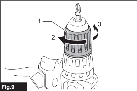
Fig.9 ► 1. Mandril 2. Cerrar 3. Abrir
